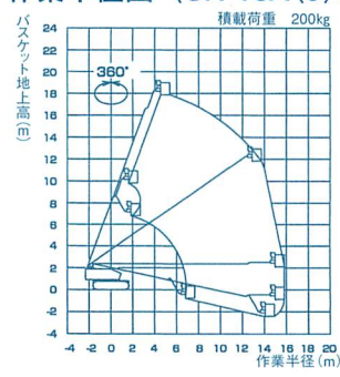
作業半径図 (SR-18A(J))
